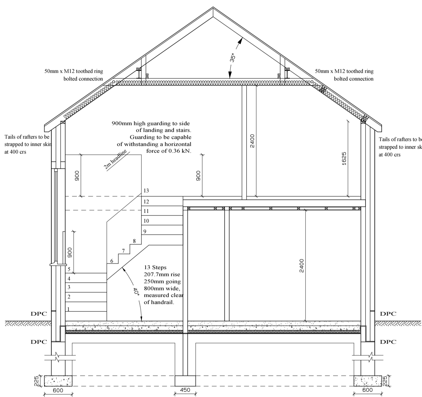
Section D-D
