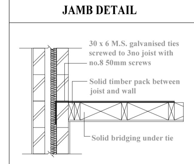
JAMB DETAIL
